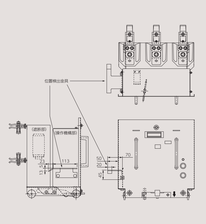
遮断器 位置検出金具取付位置
