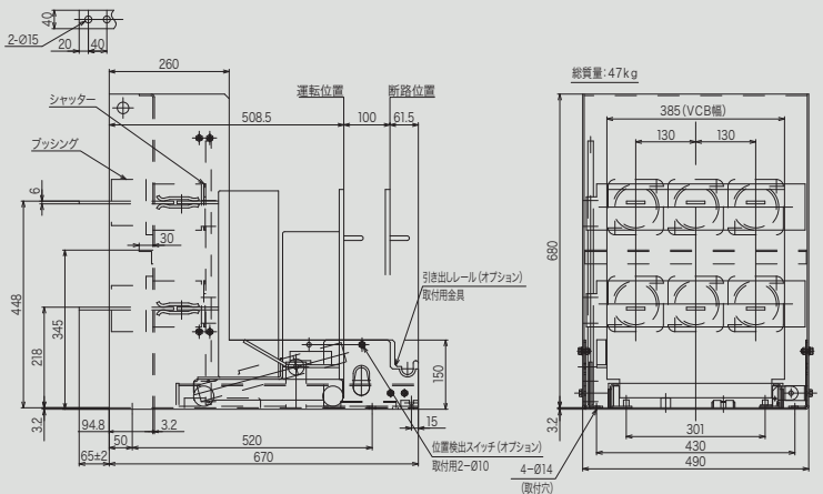
■遮断器固定枠外形寸法図
