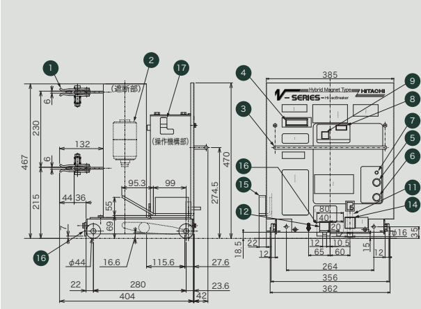
■遮断器外形寸法図
