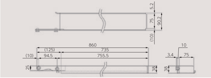
引出しレール (正面左側) 外形寸法 ※正面右側は左右対称構造 (単位：mm)
