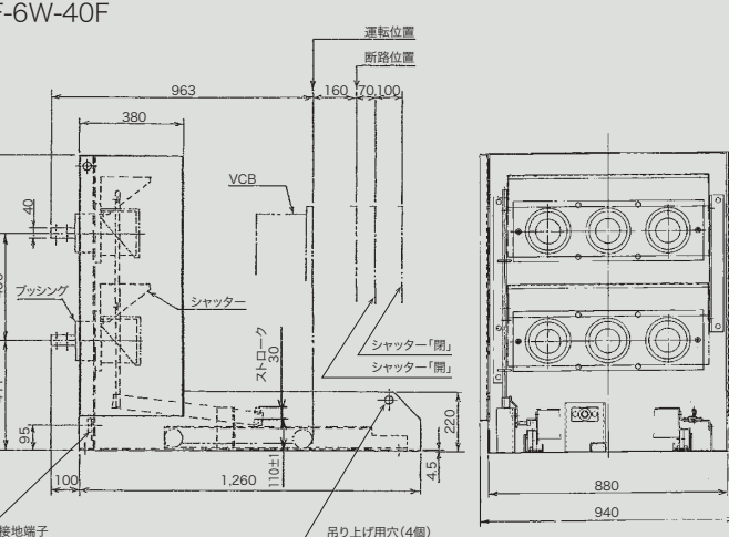
■遮断器固定枠外形寸法図
