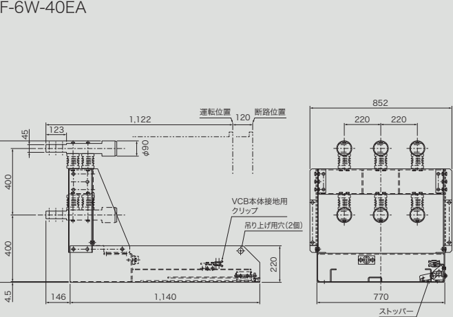
■遮断器固定枠外形寸法図
