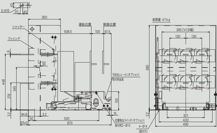
■遮断器固定枠外形寸法図
