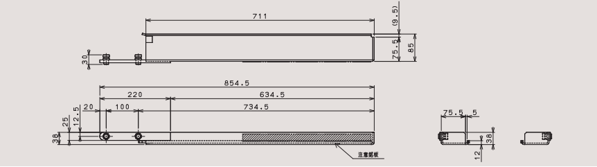
引出しレール (正面左側) 外形寸法 ※正面右側は左右対称構造 (単位：mm)
