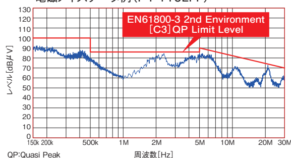
電磁ノイズデータ例 (P1-110LFF)
